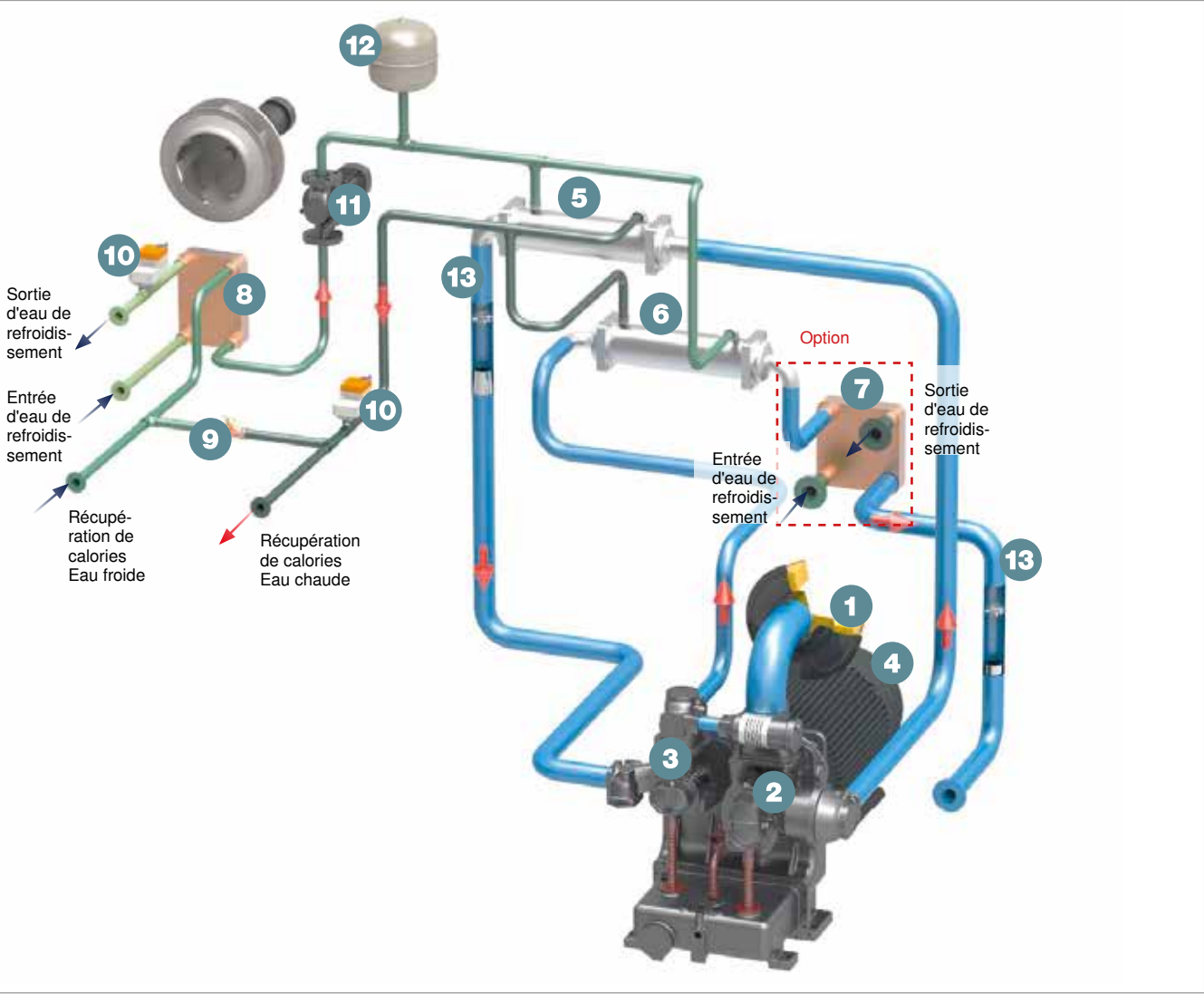
CSG refroidi par eau avec récupération des calories
