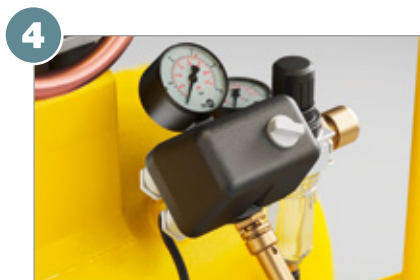
Pressostat avec démarrage à vide
